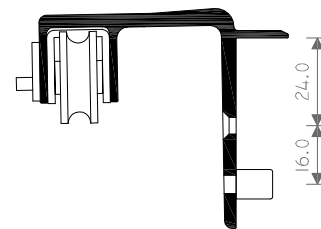
SEZIONE / SECTION / SEKTION / SECCIÓN 1:2
